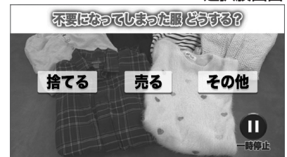
選択肢画面
